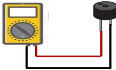
Gambar 8. Pengukuran Tegangan Buzzer
